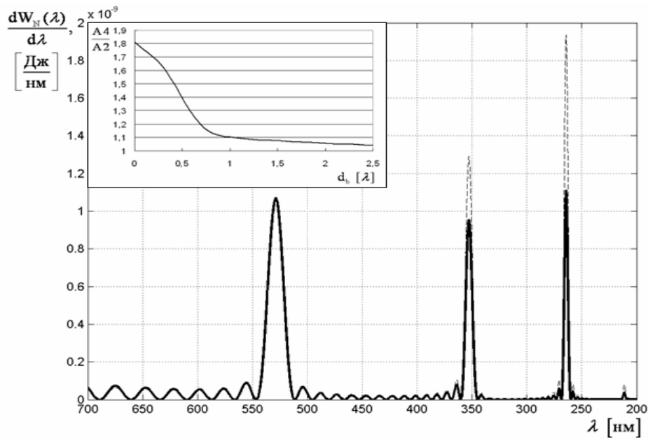
Рис.2. Вверху: Влияние размытия границы на спектр переходного излучения. Пунктирная кривая соответствует резкой границе, жирная сплошная кривая – плавной границе, d_b = 2.5 \lambda_L – длина размытия, где \lambda_L – длина волны лазерного излучения. На врезке показана зависимость отношения амплитуд четвертой и второй гармоник как функция масштаба неоднородности границы. Внизу: Влияние амбиполярного поля на спектр переходного излучения. Серая кривая соответствует нулевому полю, черная - полю с длиной торможения d_a = 0.012 \lambda_L . На врезке показана зависимость отношения амплитуды четвертой гармоники к амплитуде второй от величины амбиполярного поля
